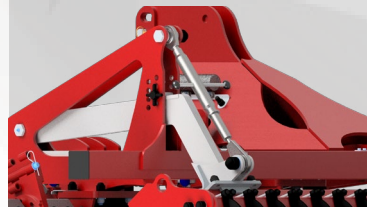
Verstellbare Scheibenreihen
