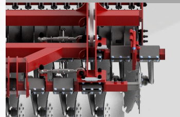
Verstellbare Scheibenreihen
