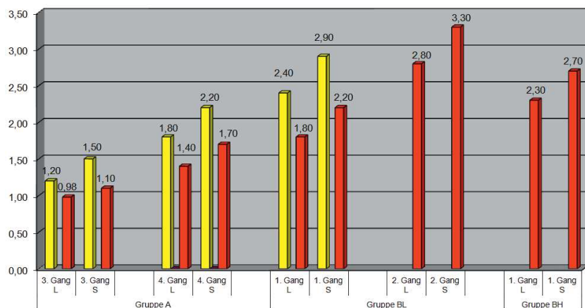
CASE Quantum 90 F Hopfen mit Ber. 340/65 R 20, 480/70 R 28 Geschwindigkeiten bei Zapfwelldrehzahl 540/750
